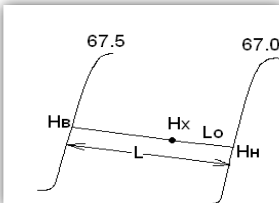
Рисунок 1 – Интерполяция
